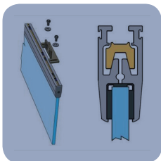
Detalle pinza
