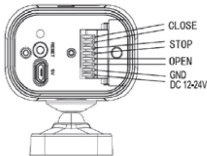
Esquema de conexiones
